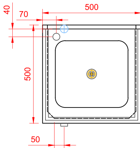
Vista Superior
